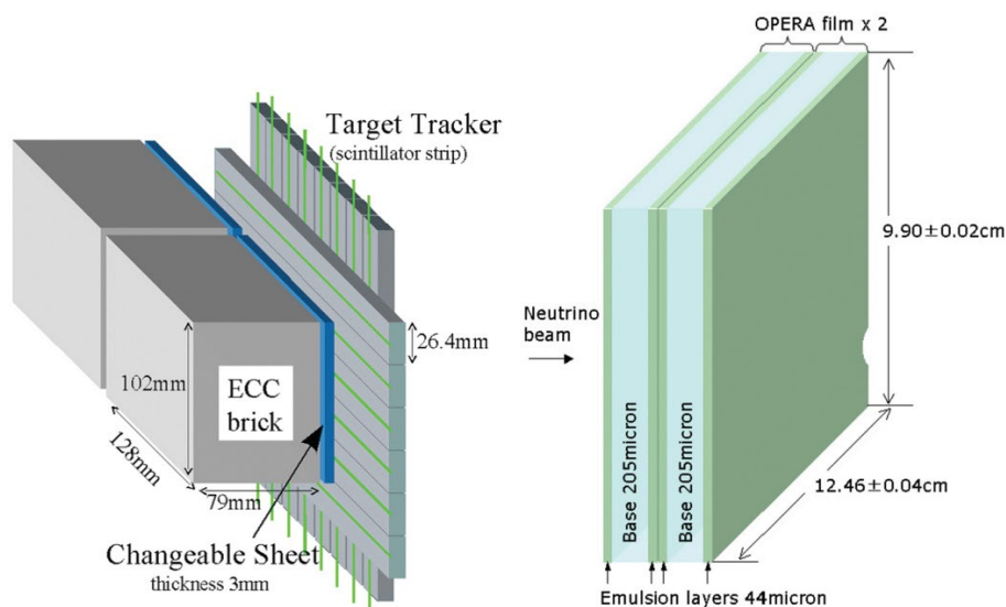
Рисунок 1.7 – Схематический вид блока ЕСС (кирпича), использованного в эксперименте OPERA. Также показана деталь сменного эмульсионного дублета
