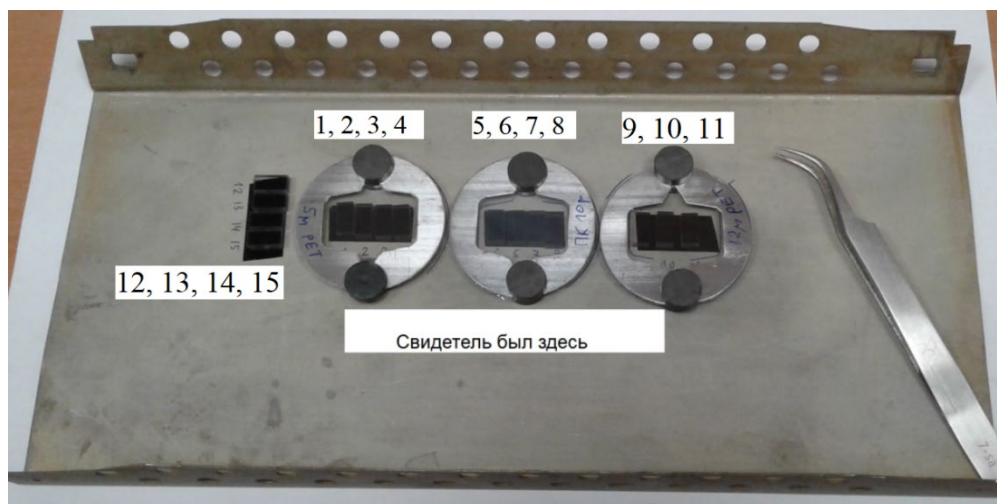
Рисунок 3.13 – Подготовленные для облучения 15 образцов стекла КНФС-3.
