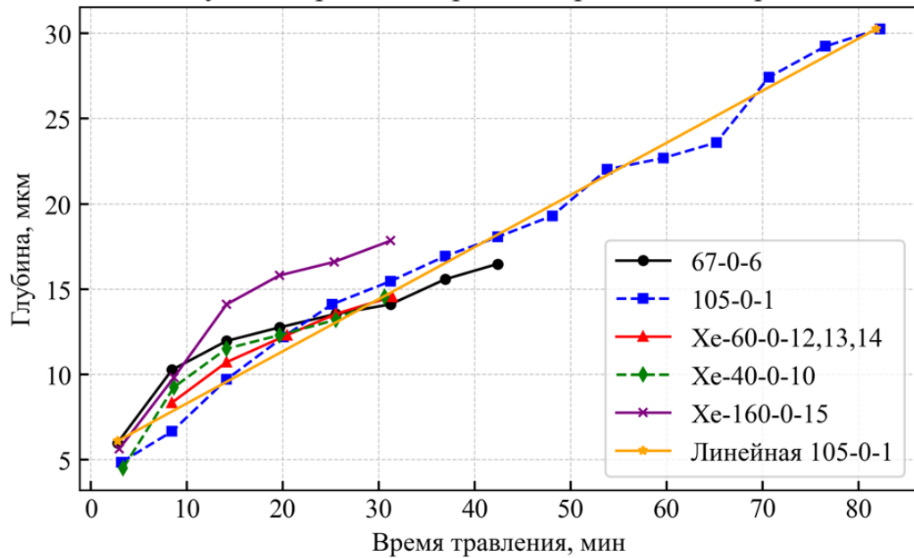
Зависимость глубины треков от времени травления. Нормальное падение
