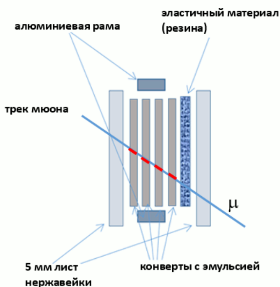
Рисунок 4.3 – Схема эмульсионного детектора.
