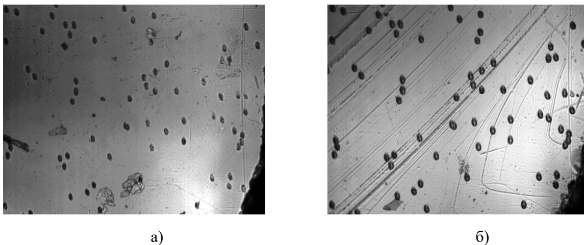
Рисунок 3.4 – Изображения поверхности одного из образцов второй группы после травления в гидроксиде натрия в течение а) 7 часов, б) 9 часов. Изображения получены на микроскопе комплекса ПАВИКОМ с объективом 20 × . Размер поля зрения 555 \times 444 мкм.
