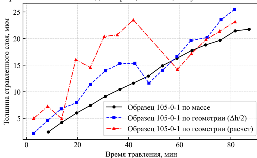
Рисунок 3.8 – Сравнительные результаты разных способов определения толщины стравленного слоя в HF
