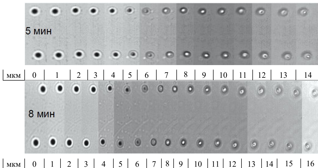
а) Вертикальное падение, энергия ионов Хе E=65-68 МэВ.
