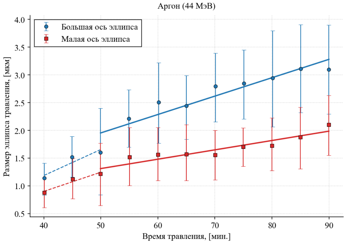
Рисунок 3.21 – Зависимость большой и малой осей эллипса на поверхности стекла от продолжительности травления для различных ионов ((а) — аргона, (б) — криптона и (в) — ксенона). Угол наклона луча к поверхности стекла составляет 30^\circ .
