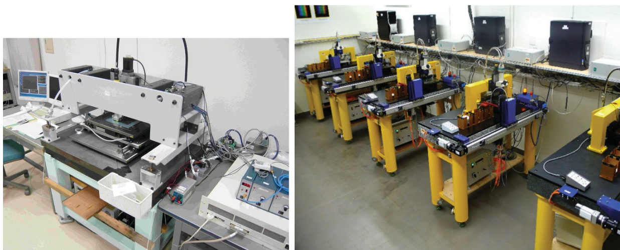
Рисунок 1.11 – Слева: Одна из сканирующих систем Nagoya S-UTS; справа: сканирующая станция в Берне, оснащенная пятью микроскопами ESS с автоматическими устройствами смены пленки.
