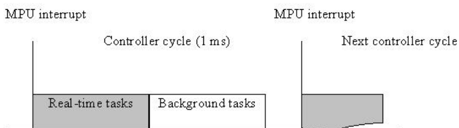
Рисунок 2.10 – Внутренняя структура цикла управления.
