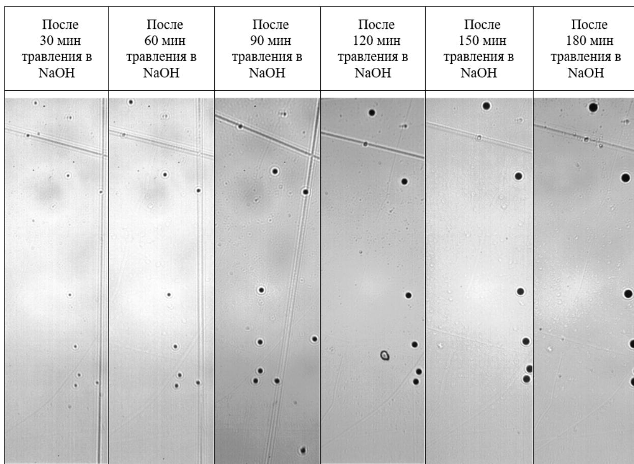
Рисунок 3.14 – Фотографии поверхности образцов КНФС-3 после травления: а) в плавиковой кислоте б) в гидроксиде натрия. Изображения получены на микроскопе комплекса ПАВИКОМ с объективом 20 х .
