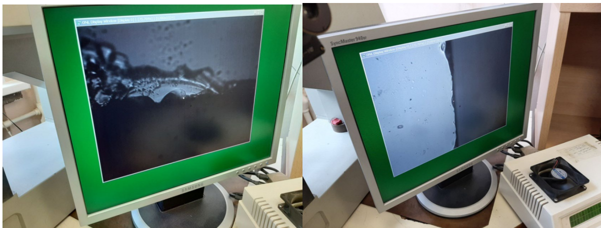
Рисунок 3.9 – Различное качество обработки граней стекол (изображение с микроскопа с объективом 40×)
