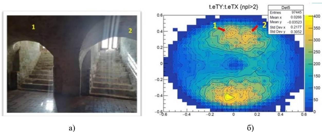
Рисунок 4.12 – Оконные проёмы в подвале ЦПБМ, «увиденные» детектором 5: а – фотография оконных проёмов, б – распределение потоков мюонов в переменных tx и ty, цифрами 1 и 2 указаны «сигналы» от оконных проёмов.
