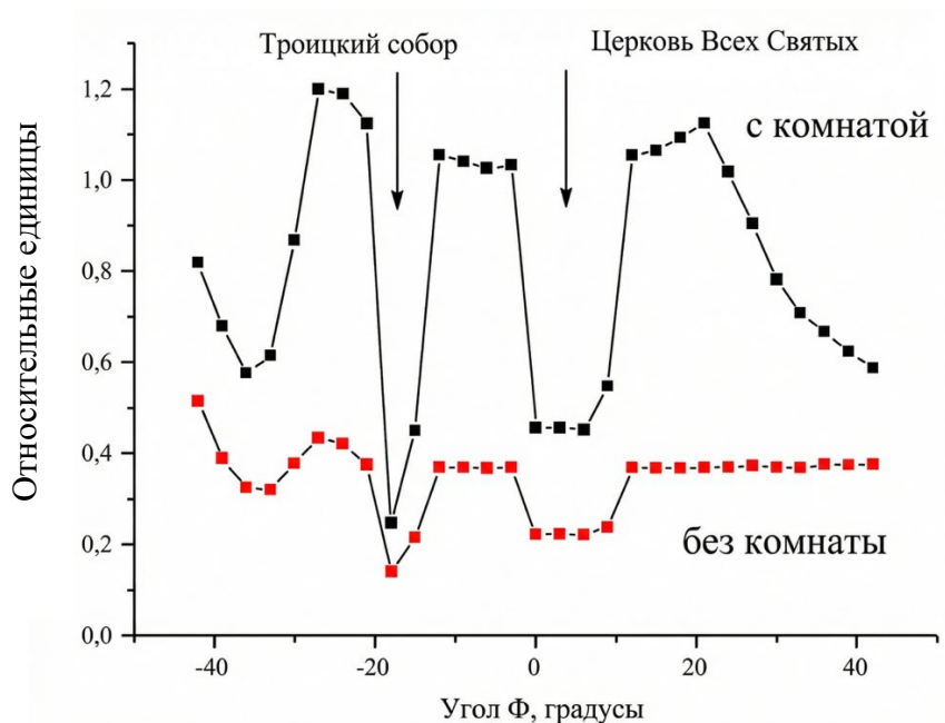
Рисунок 4.6 – Ожидаемое распределение потоков мюонов в детекторе 6 при наличии (чёрные точки) и при отсутствии (красные точки) подземной комнаты, полученное для фиксированного угла \Theta=45^\circ . Стрелками показаны «тени» от соседних зданий, образующих минимумы в распределении потоков мюонов.
