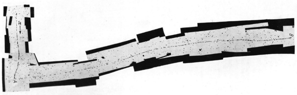
Рисунок 1.2 – Микрофотография распада \pi \rightarrow \mu , взятые из [18]
