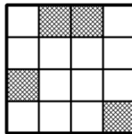
Рисунок 2.14 – Представление числа 33030 в матрице 4×4
