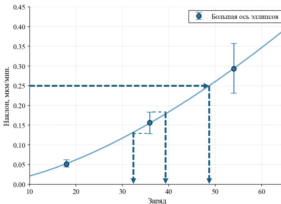
Рисунок 3.23 – Иллюстрация алгоритма определения заряда ионов.
