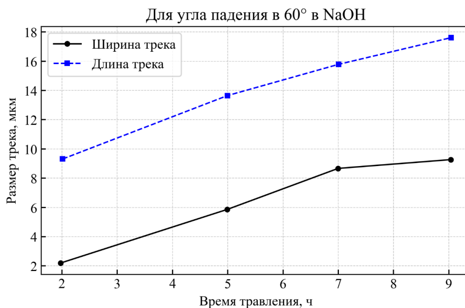
Рисунок 3.6 – Зависимость размеров протравленных треков для разных углов падения ионов от времени травления: а) диаметр в плавиковой кислоте; б) длина и ширина в гидроксиде натрия.
