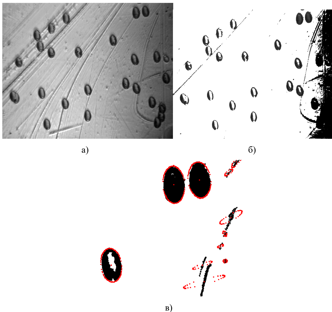
Рисунок 3.12 – Результат обработки следов ионов ^{132}\text{Xe}^{26+} с энергией 1 МэВ/А (под углом 60^\circ к нормали) после травления плавиковой кислотой в течение 9 часов: а) – исходное изображение на микроскопе; б) – результат обработки изображения с помощью разработанной программы; в) – небольшой фрагмент результата обработки. Большая ось эллипса 18 мкм, малая 11 мкм.
