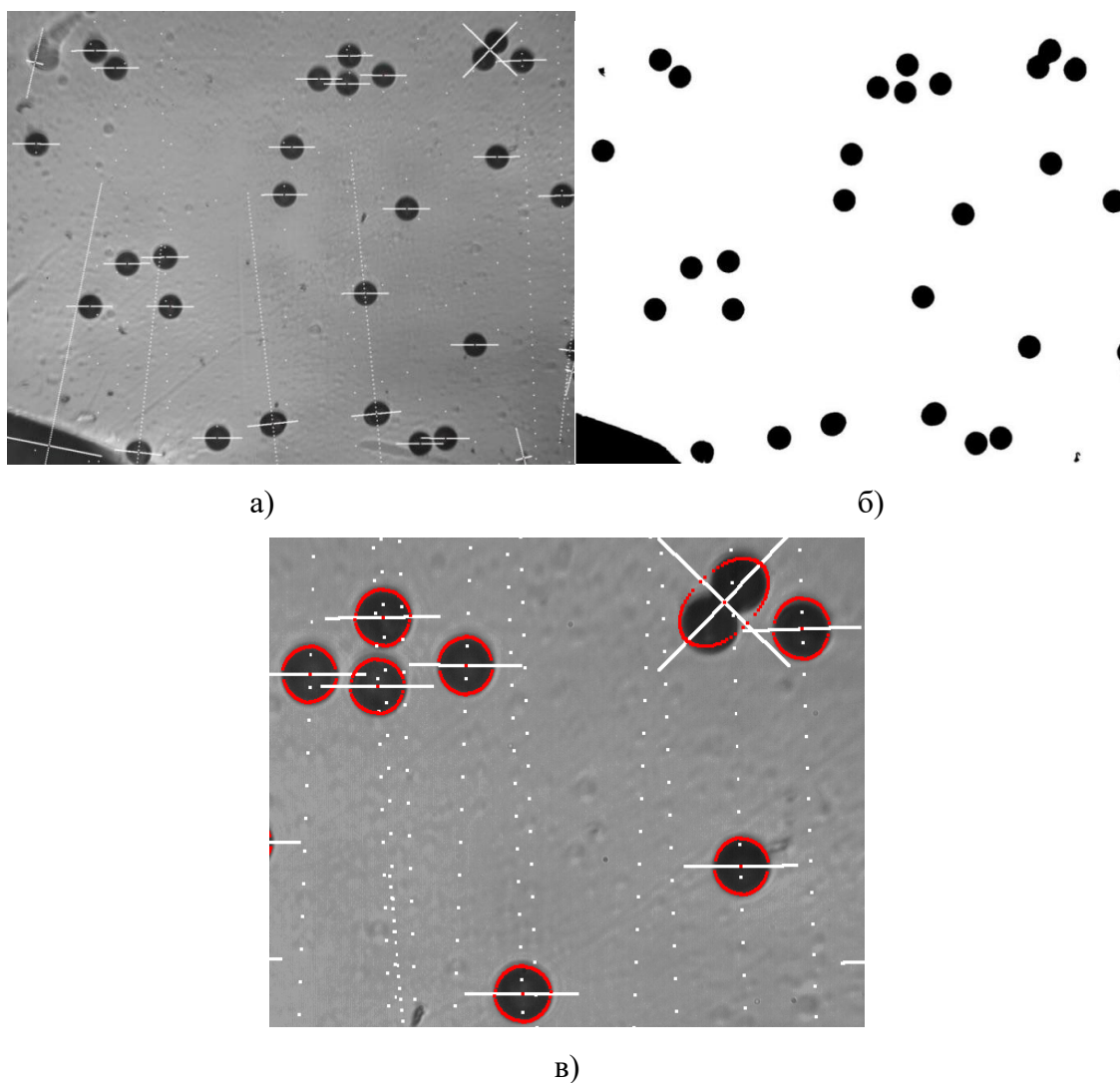
Рисунок 3.11 – Результат обработки следов ионов ^{132}\text{Xe}^{26+} с энергией 1 МэВ/А (нормальное падение, стекло ГЛС-22) после травления плавиковой кислотой в течение 20 минут: а) – исходное изображение на микроскопе; б) – результат обработки изображения с помощью разработанной программы; в) – небольшой фрагмент результата обработки.
