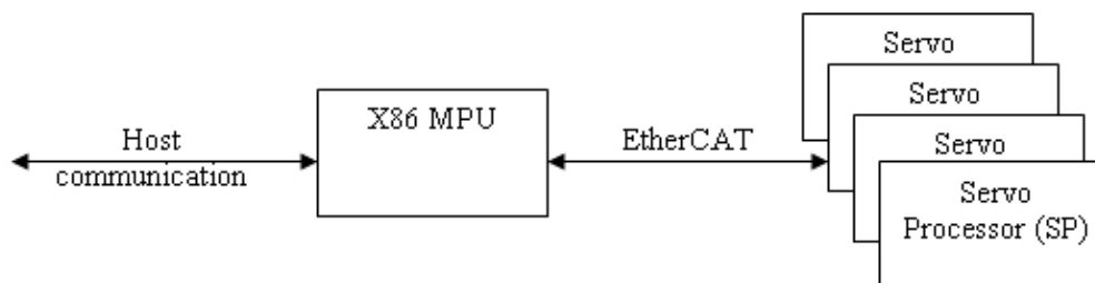
Рисунок 2.8 – Аппаратная структура контроллера SPiiPlus.
