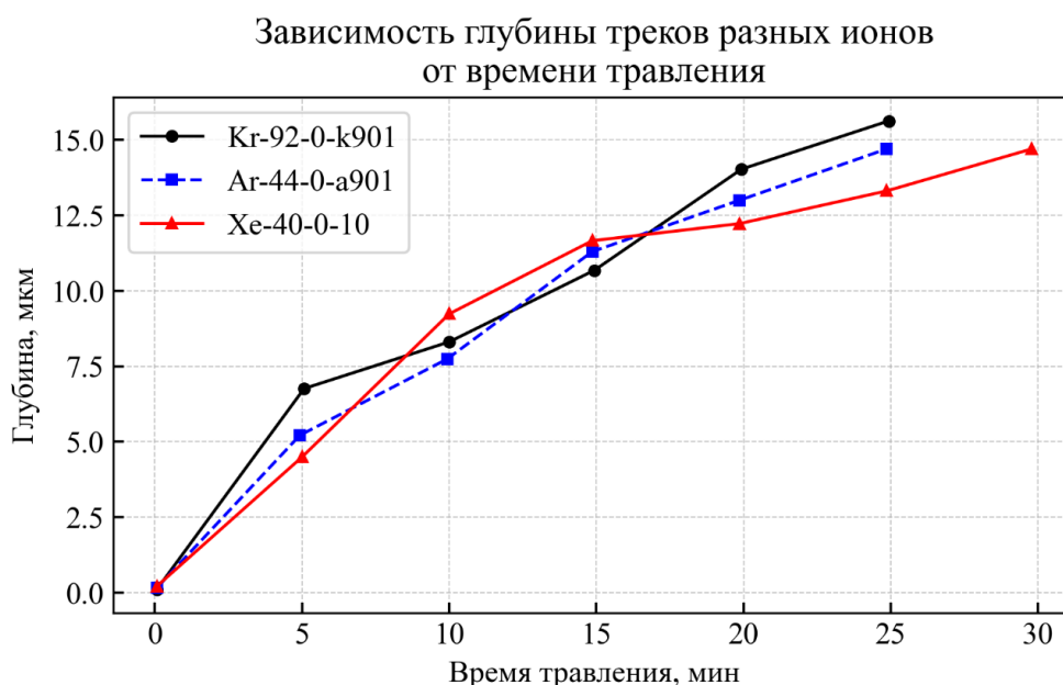
Рисунок 3.18 – Зависимость глубины треков разных ионов от времени травления.
