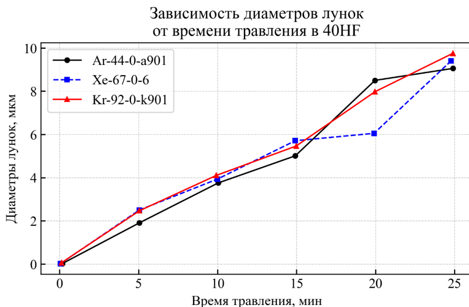
Рисунок 3.19 – Диаметры лунок от различных ядер при нормальном падении пучка.
