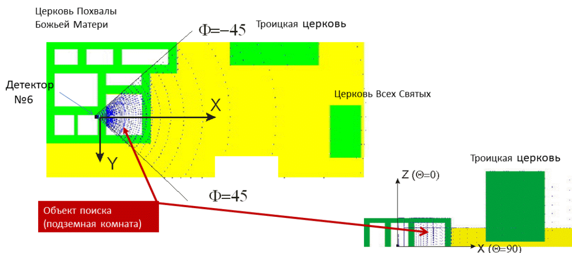
Рисунок 4.5 – Схема модельного эксперимента для детектора б (указаны направления \Phi = \pm 45^\circ ), установленного в подвале ЦПБМ. Справа от детектора под землей была добавлена скрытая комната, существование которой предполагалось на начальном этапе работ (отмечена стрелкой).
