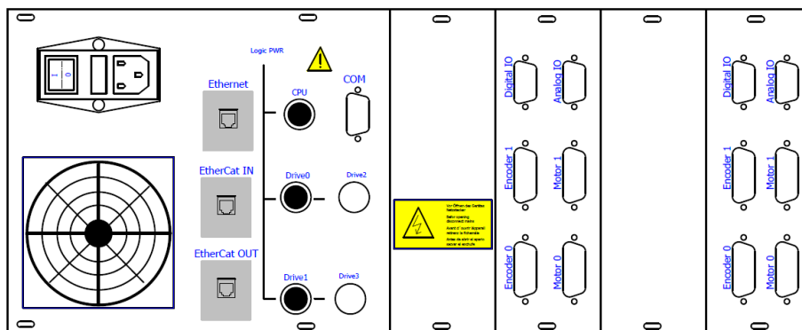
Рисунок 2.7 – Схема выводов контроллера G-900K044.
