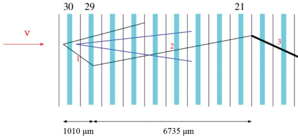
Рисунок 1.5 – Схематический рисунок первого нейтринного события рождения чарма, наблюдаемого в эмульсиях эксперимента CHORUS
