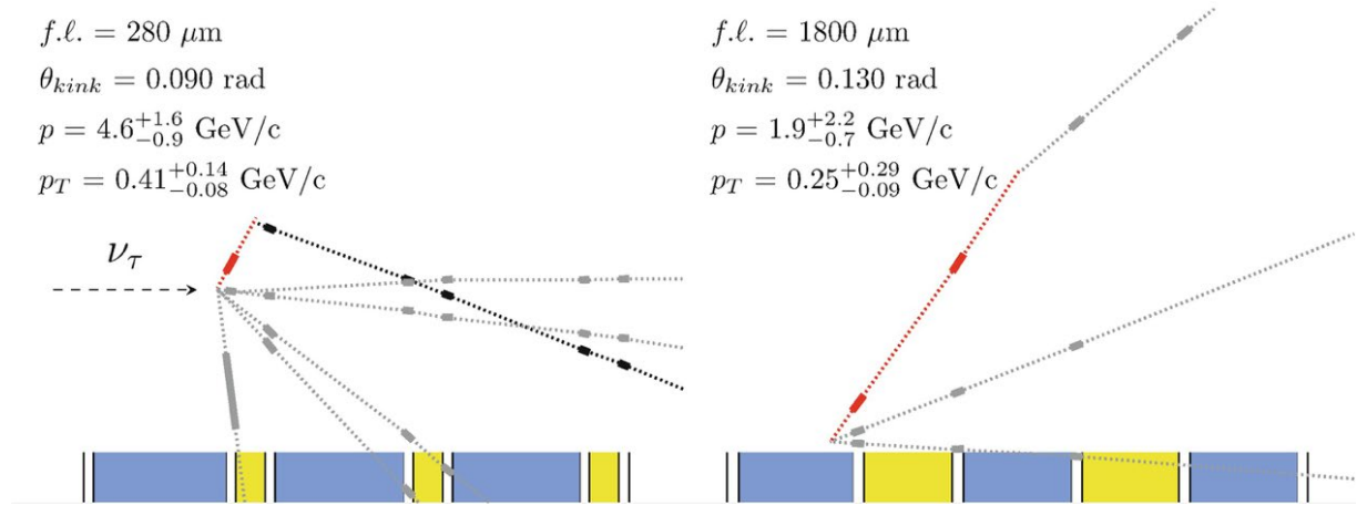
Рисунок 1.6 – Схематическое изображение двух событий, вызванных \nu_\tau , зарегистрированных в эксперименте DONUT. Видны перегибы, связанные с распадом \tau . Цветные прямоугольники внизу каждого события указывают материал: синий — сталь (основной материал мишени ECC), желтый — пластиковая подложка, белый — эмульсия.
