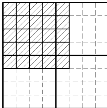
Рисунок 2.20 – Добавочные матрицы.
