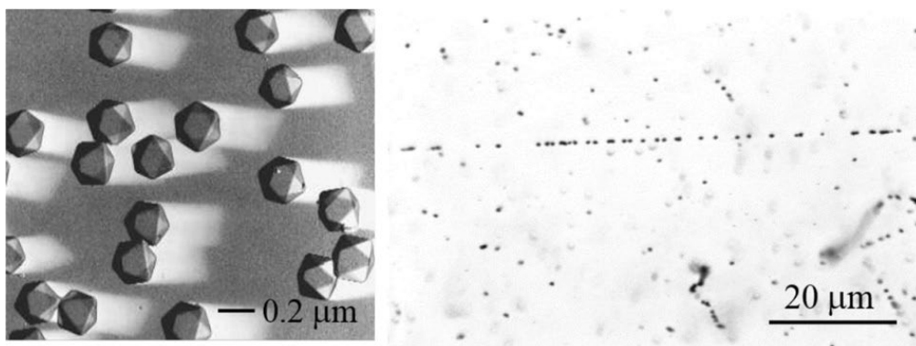
Рисунок 1.1 – Слева: кристаллы бромида серебра (линейный размер 0,2 мкм), видимые с помощью электронного микроскопа. Справа: след, оставленный минимально ионизирующей частицей ( \pi – с энергией 10 ГэВ) в ядерных эмульсиях; обнаружено около 36 зерен на 100 мкм. Комптоновские электроны с энергией приблизительно 100 кэВ также видны в правом нижнем углу изображения
