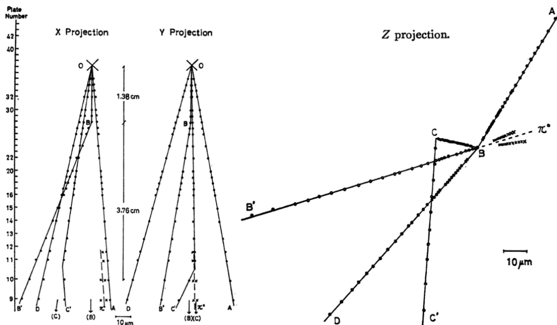
Рисунок 1.3 – Схематический рисунок первых свидетельств образования и распада короткоживущих “X-частиц” (очарованных мезонов) при взаимодействии космических лучей
