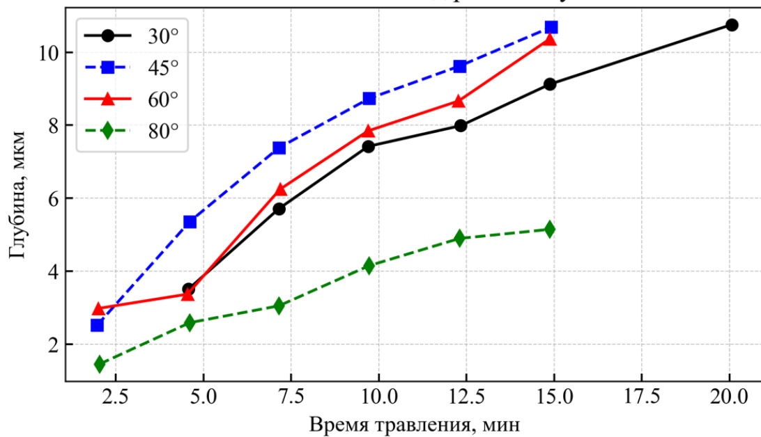
Зависимость глубины треков от времени травления Ионы Xe 160 МэВ под разными углами
