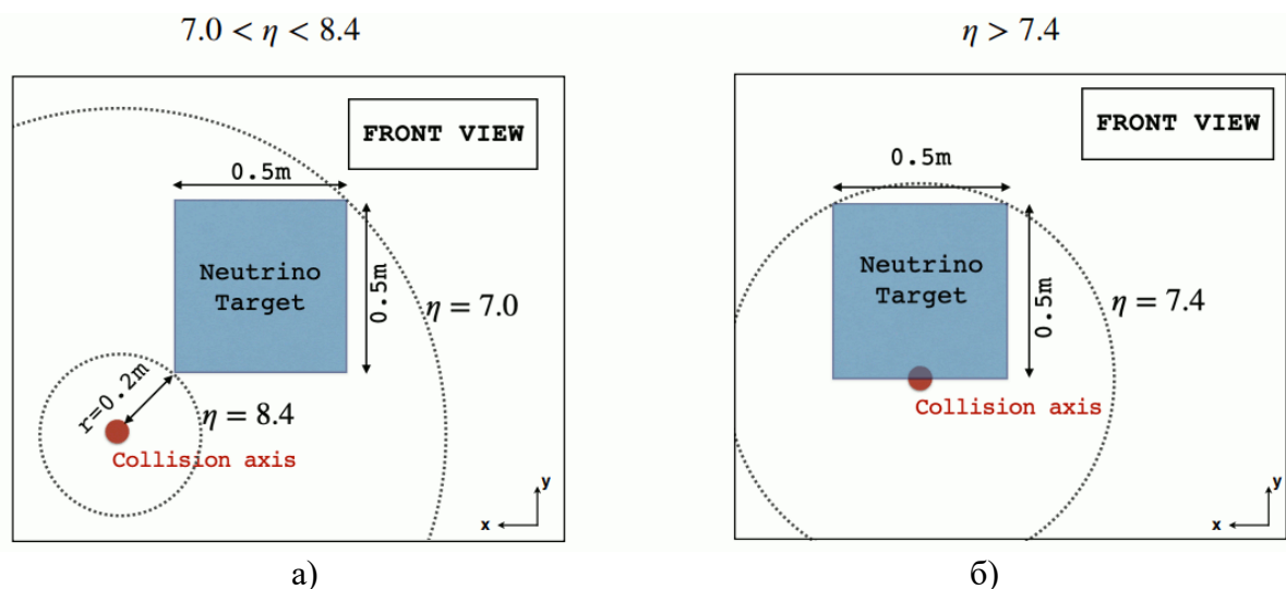
Рисунок 2.18 Схематическое изображение нейтринного детектора SND@LHC относительно оси пучка, вид спереди: а) во время экспозиций RUN1÷RUN14, б) предполагаемое положение при последующих экспозициях [43].
