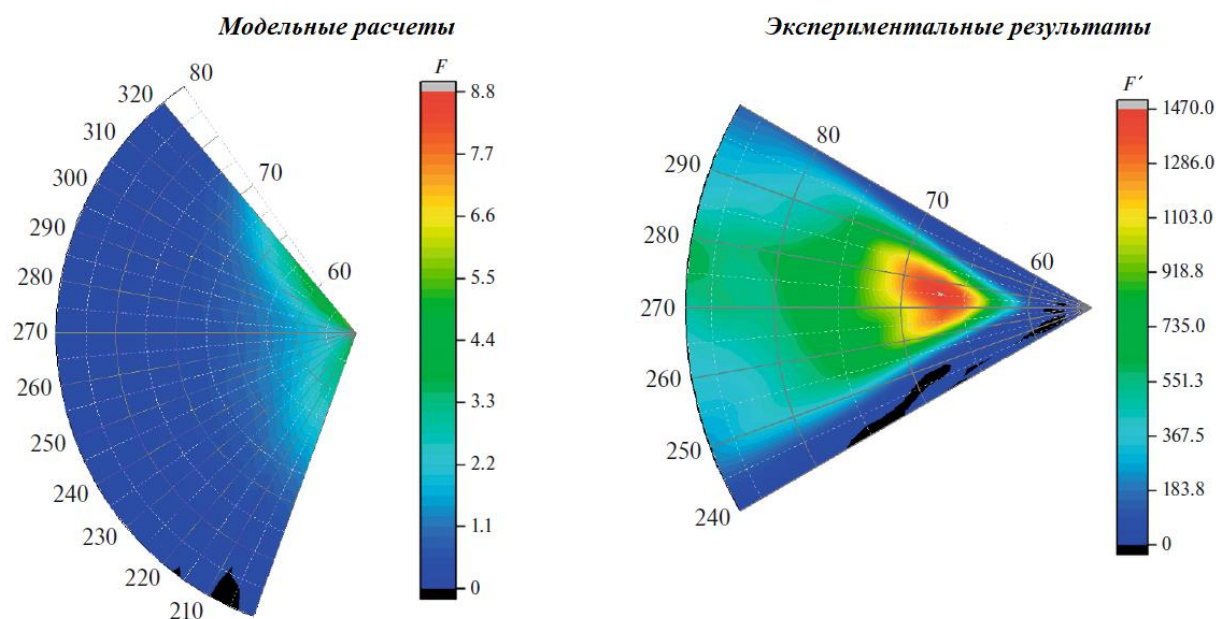
Рисунок 4.65 Распределение числа частиц в элементе телесного угла ( \Delta\varphi , \Delta\theta ) как функция углов \varphi и \theta для детектора №2 в прямом направлении для модельных расчетов F(\varphi, \theta) и экспериментальных результатов F'(\varphi, \theta) . Радиусы соответствуют линиям постоянства угла \varphi , а дуги — линиям постоянства угла \theta . Цветная вертикальная шкала отображает число зарегистрированных мюонов.
