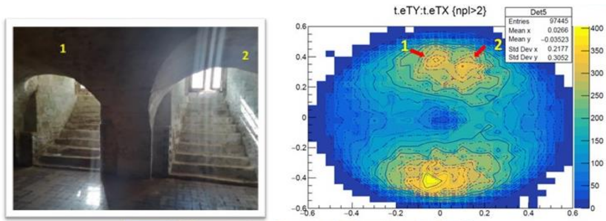
Рисунок 10 – Оконные проёмы в подвале ЦПБМ, «увиденные» детектором 5: а – фотография оконных проёмов, б – распределение потоков мюонов в переменных t_x и t_y , цифрами 1 и 2 указаны «сигналы» от оконных проёмов.
