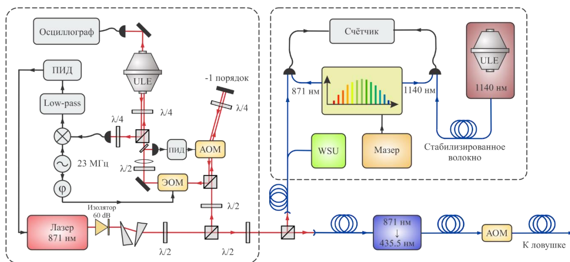
Рисунок 4.6 – Схема высокостабильной лазерной системы на длине волны 435.5 нм, а также установки для характеристики ее стабильности. WSU – измеритель длин волн, ЭОМ – электрооптический модулятор, АОМ – акустооптический модулятор. Кубиками обозначены поляризационные светоделители.
