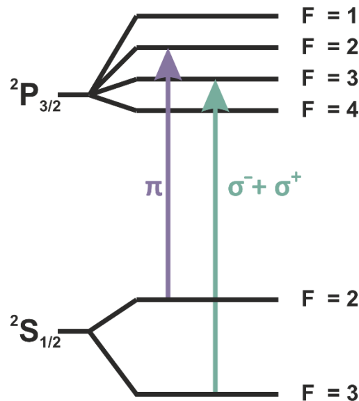
Рисунок 3.4 – Схема оптической накачки иона магния в состояние {}^2S_{1/2}(F=2, m_F=0) . Символами \pi, \sigma^+, \sigma^- обозначены поляризации соответствующих пучков.
