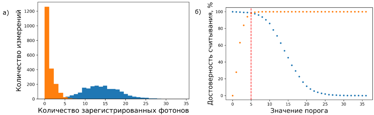
Рисунок 4.11 – а) Гистограмма отсчетов, зарегистрированная ФЭУ когда ион в светлом состоянии (синие столбцы) и когда флуоресценция иона подавлена (оранжевые столбцы, симуляция иона в темном состоянии). б) Зависимость достоверности детектирования темного (оранжевые точки) и светлого (синие точки) состояний в зависимости от порогового значения дискриминатора. Пунктирной линией отмечено оптимальное значение, равное 5.
